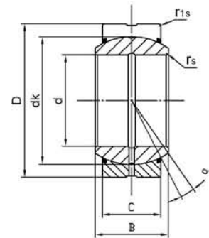
GEZ..ES-2RS
