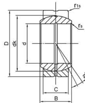
GEZ..ES
