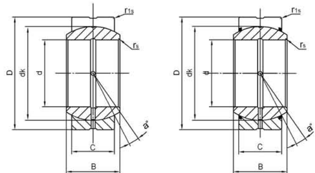
GEZ..ES
