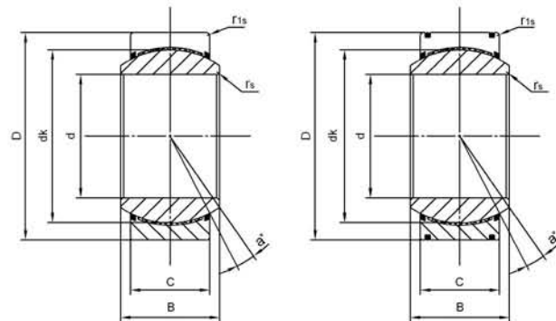
GEG..ET-2RS
