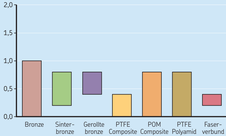
Oberflächenrauheit der Welle R_a, \mu\text{m}
